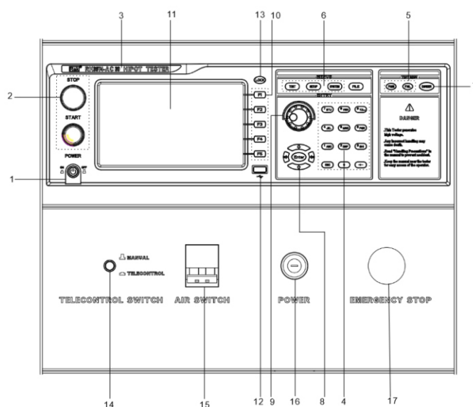
图3.5 前面板说明
