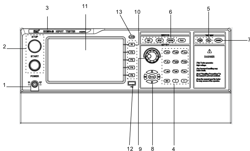
图 3-3前面板说明
