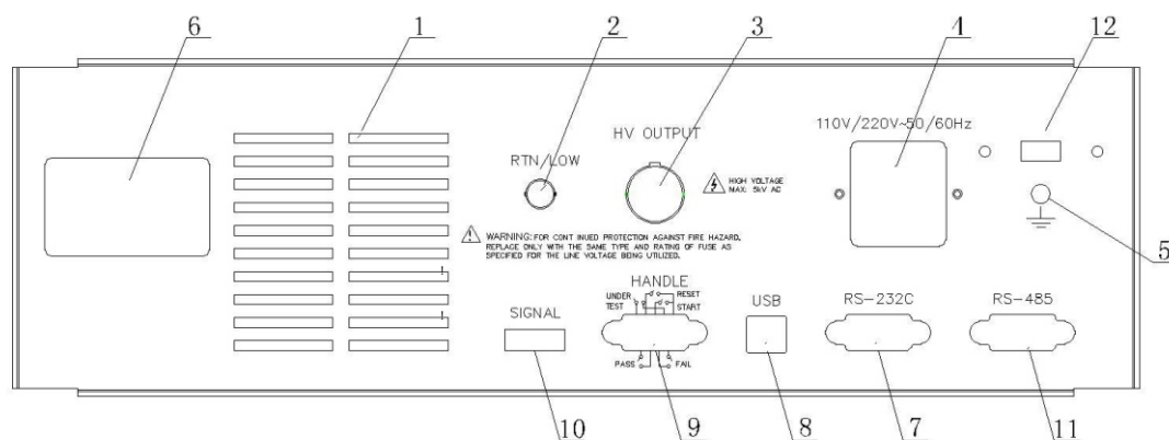
图 3-2 后面板说明
