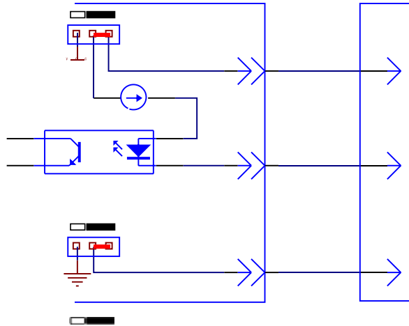
图 7-2 输入信号简化示意图
