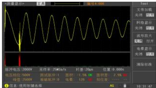
图 4-5 波形正常显示时的电晕显示
