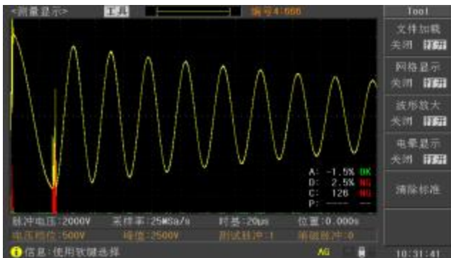
图 4-4 波形放大显示时的电晕显示
