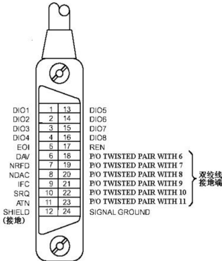
图 5-2 GPIB 接插件/管脚结构图
