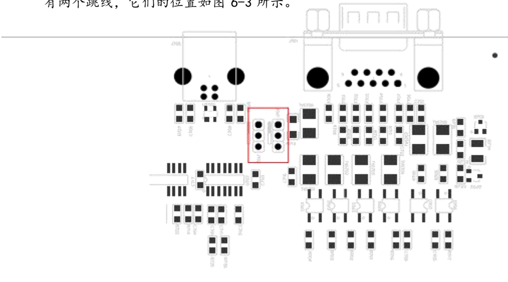
图 6-3 跳线在 Handler 板上的位置
