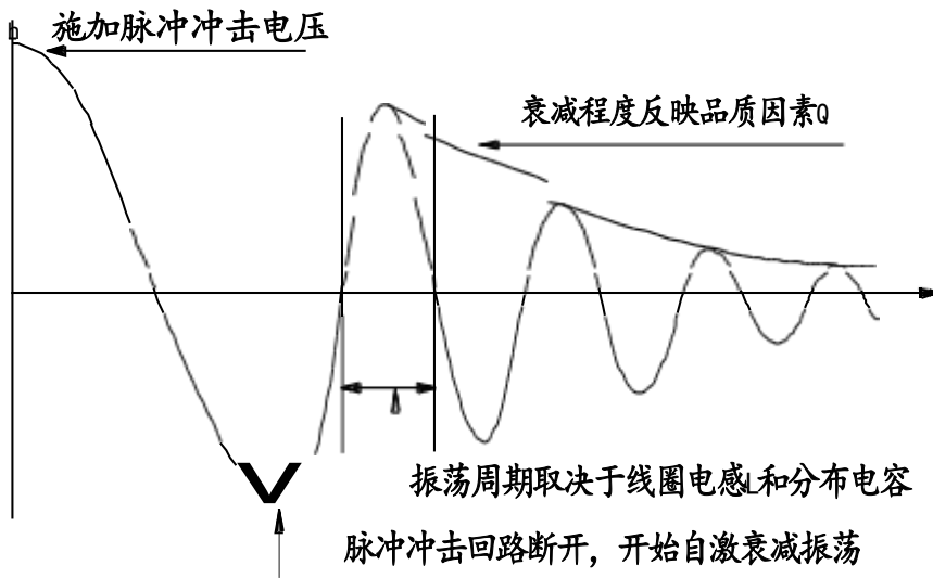
图 1-2 典型的线圈自激衰减振荡波形
