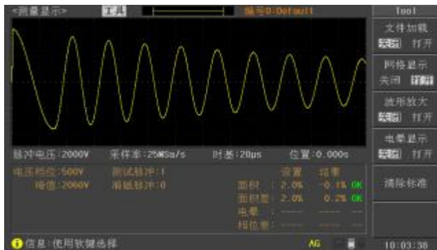
图 4-2 波形正常显示
