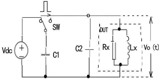
图 1-1 线圈脉冲测试原理简图
