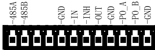
图 5-2 RS485 串口
